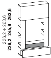
modulo tv multimedia multimedia tv module
