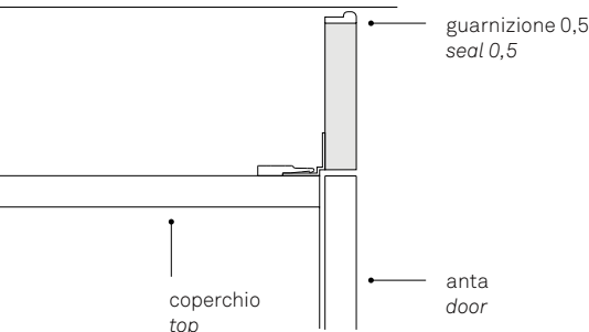
posizionamento superiore upper positioning
