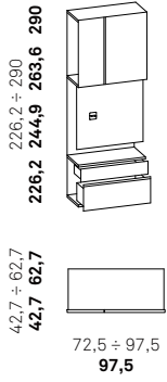
modulo porta tv apribile opening tv module
