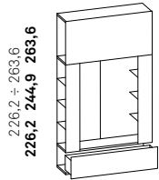
modulo tv tv module
