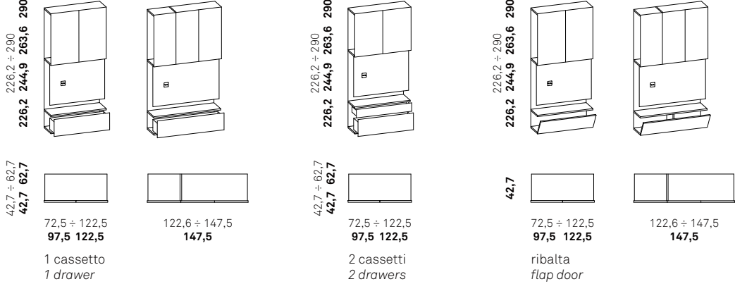
modulo porta tv apribile opening tv module
