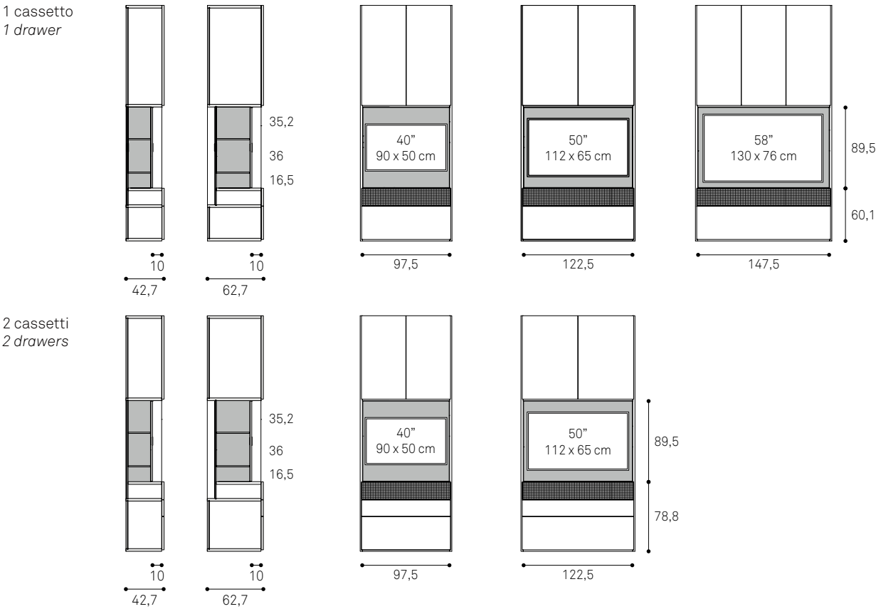
modulo porta tv apribile | opening tv module
