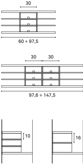
Le griglie possono essere accessoriate in base alla larghezza con i relativi vassoi rivestiti in tessuto. Grids can be accessorized with fabric-covered trays according to their width.
