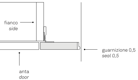
posizionamento laterale lateral positioning
