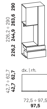
modulo portabiti a giorno open-front garment module
