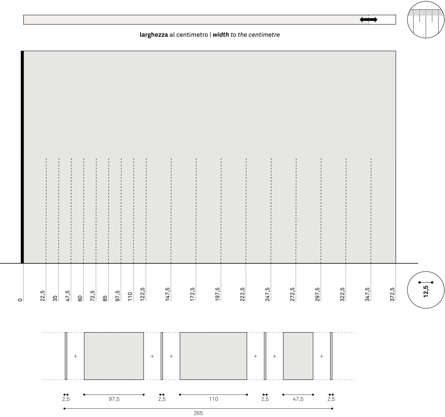
progettazione modulare modular design
