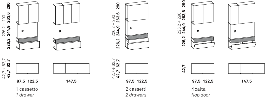
modulo porta tv apribile multimedia multimedia opening tv module
