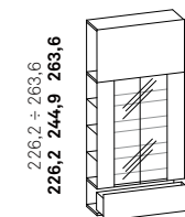
modulo vetrina showcase module
