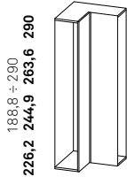
modulo angolo battente swing door corner module
