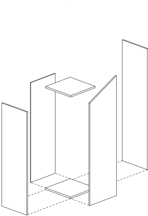
anta battente (no vetro-specchio) - cabina swing door (no glass-mirror) - cabina
